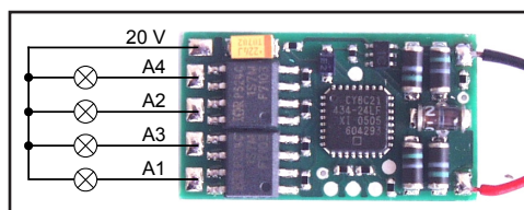
Die beiden Möglichkeiten den Decoder anzuschliessen
